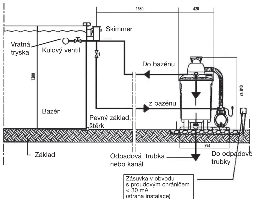
obr. 5 Příklad instalace
